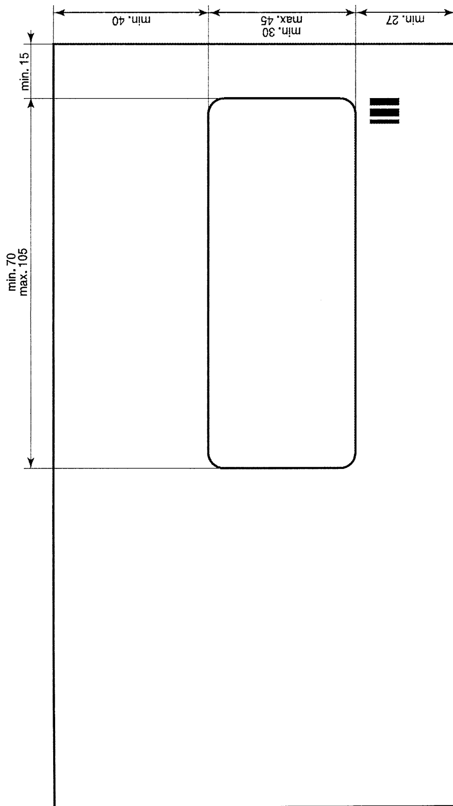
Obrázek 7 - Okénková obálka v provedení s okénkem v pravé části adresní strany
